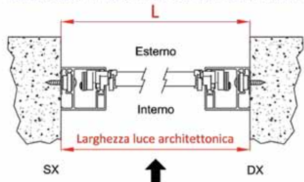
SEZ. ORIZZONTALE X-X CON GUIDE NON INCASSATE
