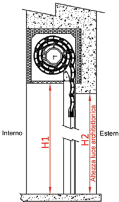
SEZ. VERTICALE Y-Y CON TELO AVVOLTO
