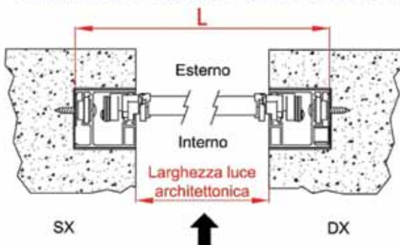
SEZ. ORIZZONTALE X-X CON GUIDE INCASSATE
